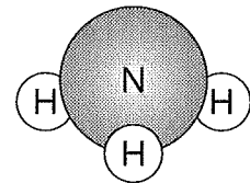
アンモニア \text{NH}_3
