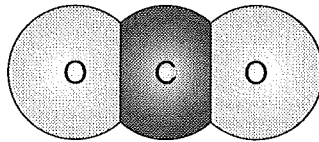
二酸化炭素 \text{CO}_2
