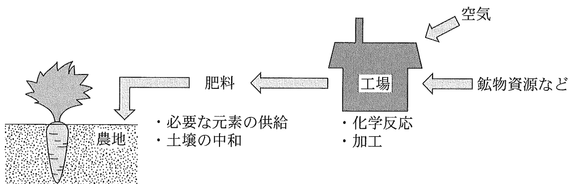
図1 鉱物資源などを原料とする肥料の利用
