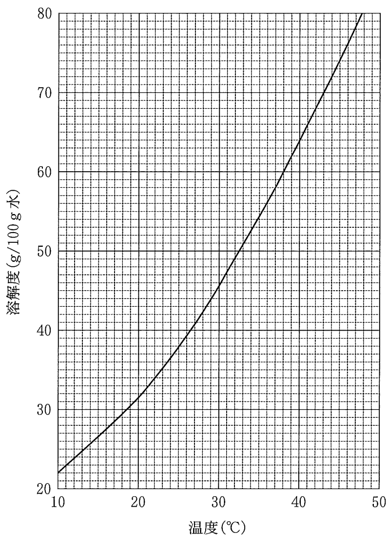
図 2 \text{KNO}_3 の水に対する溶解度曲線
